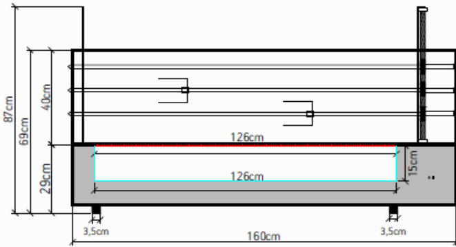
VISTA LATERAL
