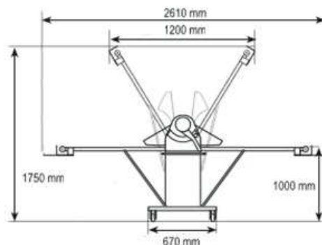
VISTA LATERAL
