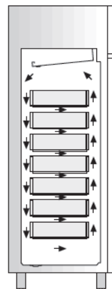
CIRCULAÇÃO DO FLUXO DE AR INTERIOR
